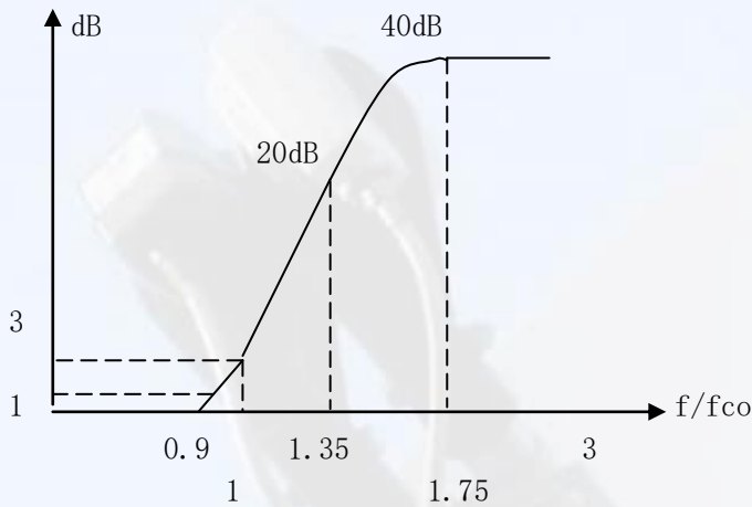
典型的低通频响特性
